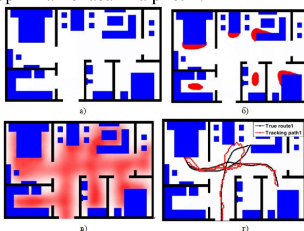
Рисунок 1 - Результаты обработки измерений тепловыми датчиками: а) исходный план помещения, б) места стационарного размещения человека, в) тепловая карта перемещения по помещению, г) вычисленная траектория перемещения человека
