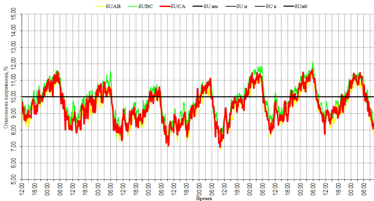
Рисунок 2 – Недельный график отклонения междуфазных напряжений
