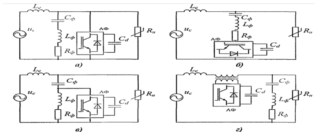
Рисунок 3 – Варианты гибридных фильтров с параллельным и последовательным подключением силового электронного регулятора относительно сети
