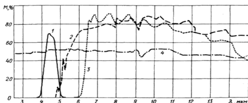
Рисунок 3 - Различные спектральные характеристики пироэлектрических датчиков. 1 – для обнаружения пламени; 2,3 – для фиксации движения человека; 4 – для использования в дистанционных измерителях температуры
