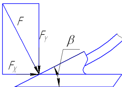
Рисунок 2 – Силы, приложенные к лапе культиватора
