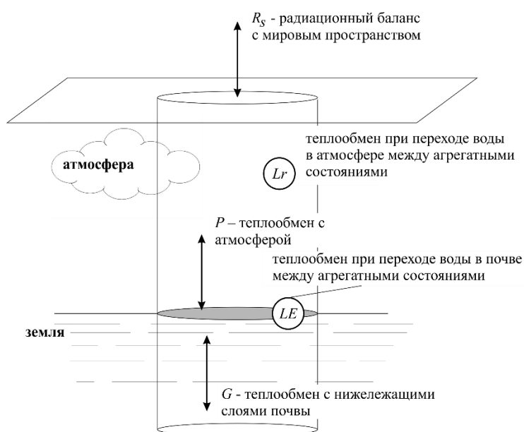
Рисунок 1 - Модель теплового баланса системы земля-атмосфера
